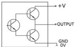
Totempole output
