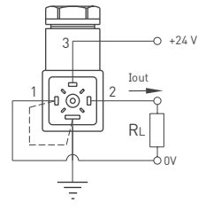
0-20mA or 4-20mA Output
